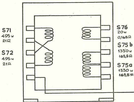
VOEDING TRAF0 GK 512 62
